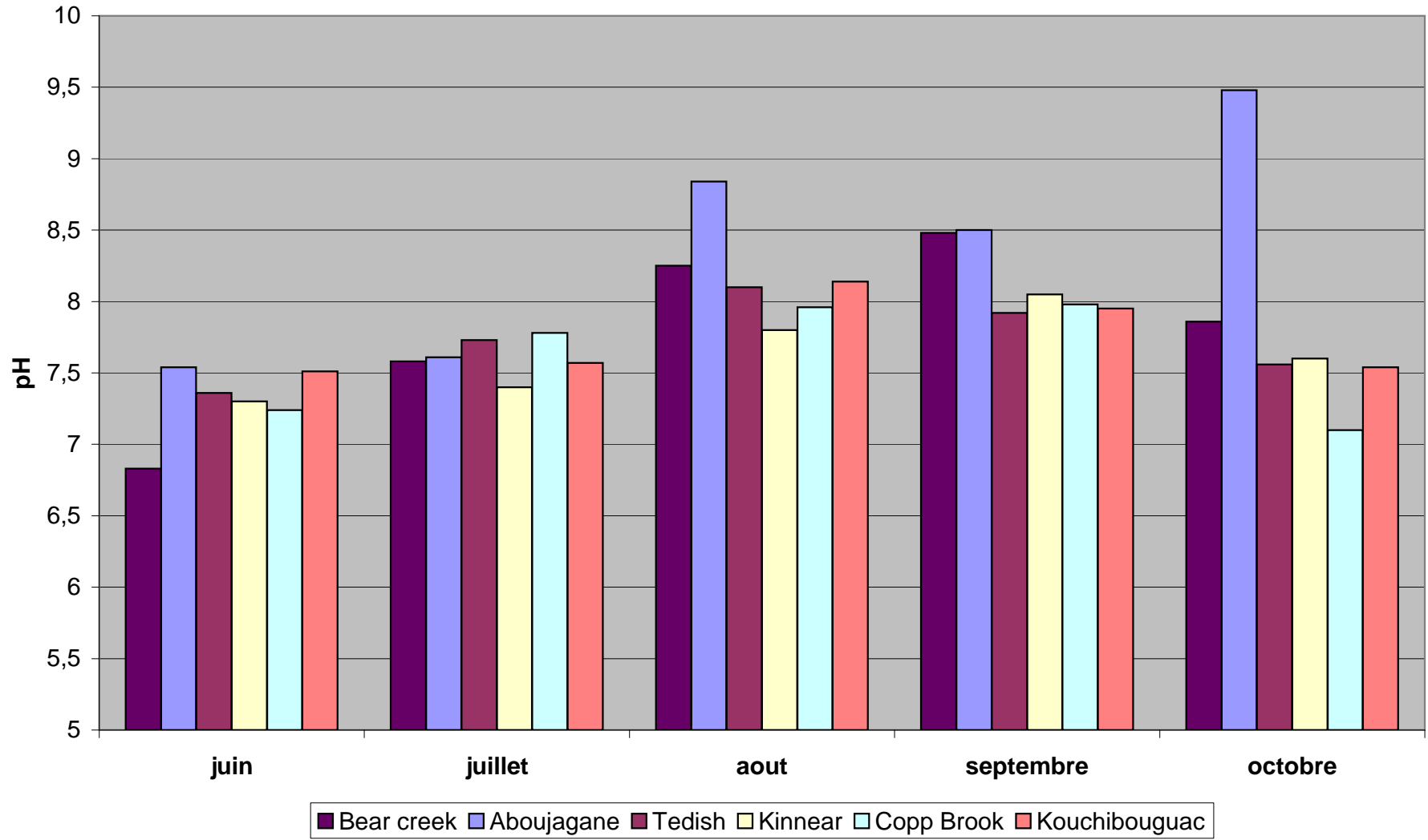
pH mensuel mesuré au six site d'échantillonnage (2007)
